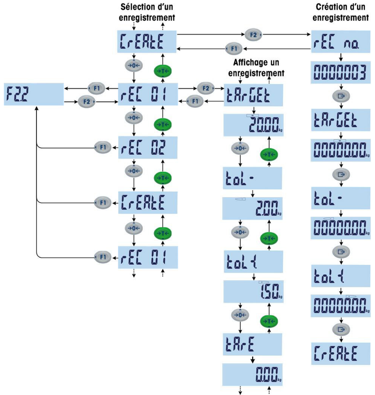
Figure 3-42 : Sélection, Examen et Création d'enregistrements
